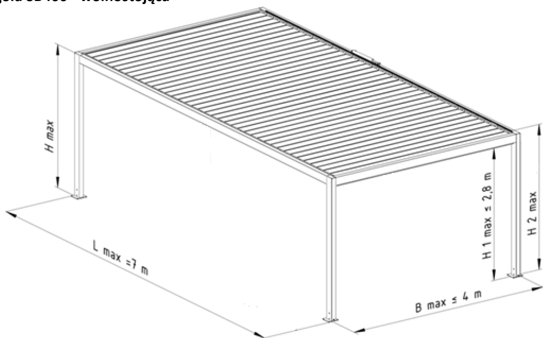
Rys. 1. Pergola SB400 wolnostojąca - Wymiary gabarytowe: B max – szerokość maksymalna, L max – długość maksymalna, H max – wysokość maksymalna ramy (3012 mm), H 1 max – prześwit w świetle ramy, H 2 max – wysokość maksymalna położenia mechanizmu zmiany kąta piór (~3140 mm).
