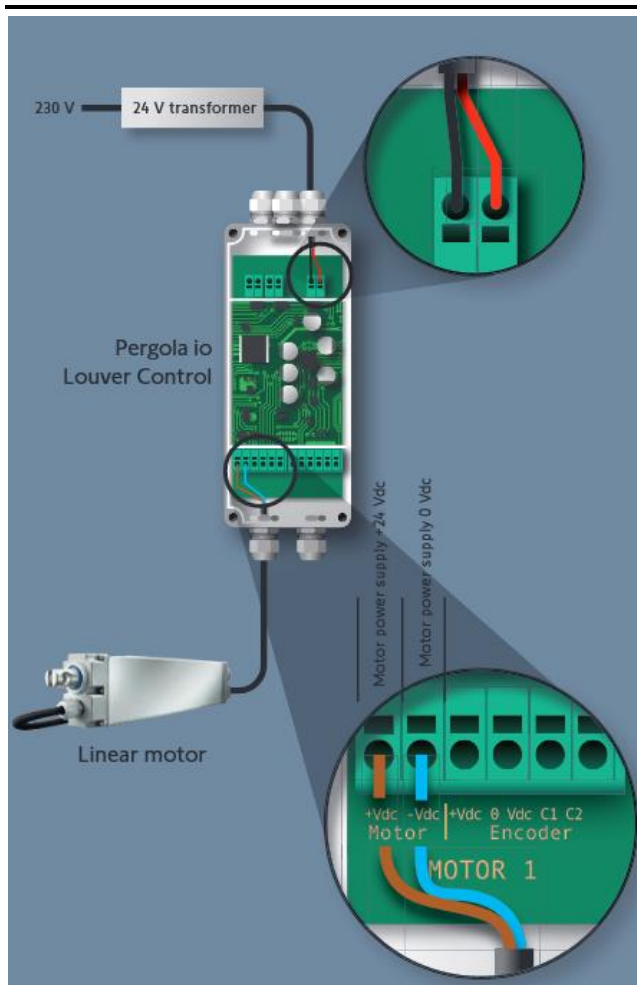
Rys. 65 Schemat obszarów podłączeń wewnątrz centralki Pergola io Louver Control (opisy na dolnym powiększeniu podano jako pogrubione w tabeli powyżej)
